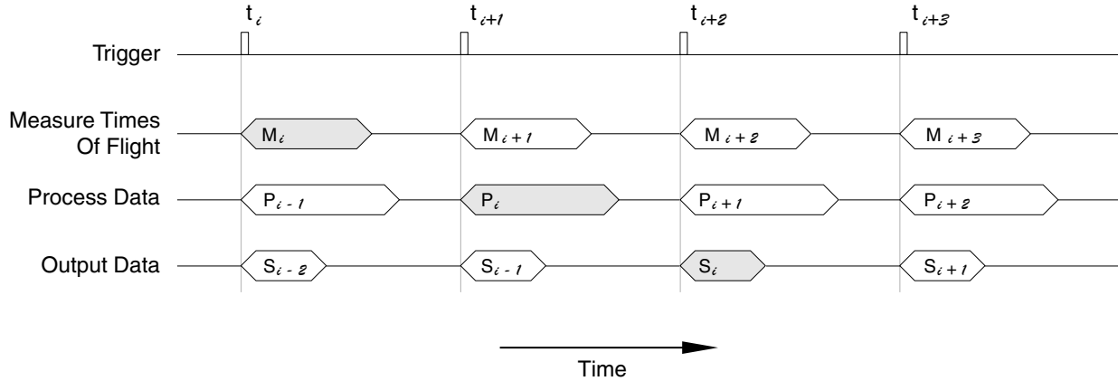
FIGURE 5. CSAT3 Pipeline Delay
